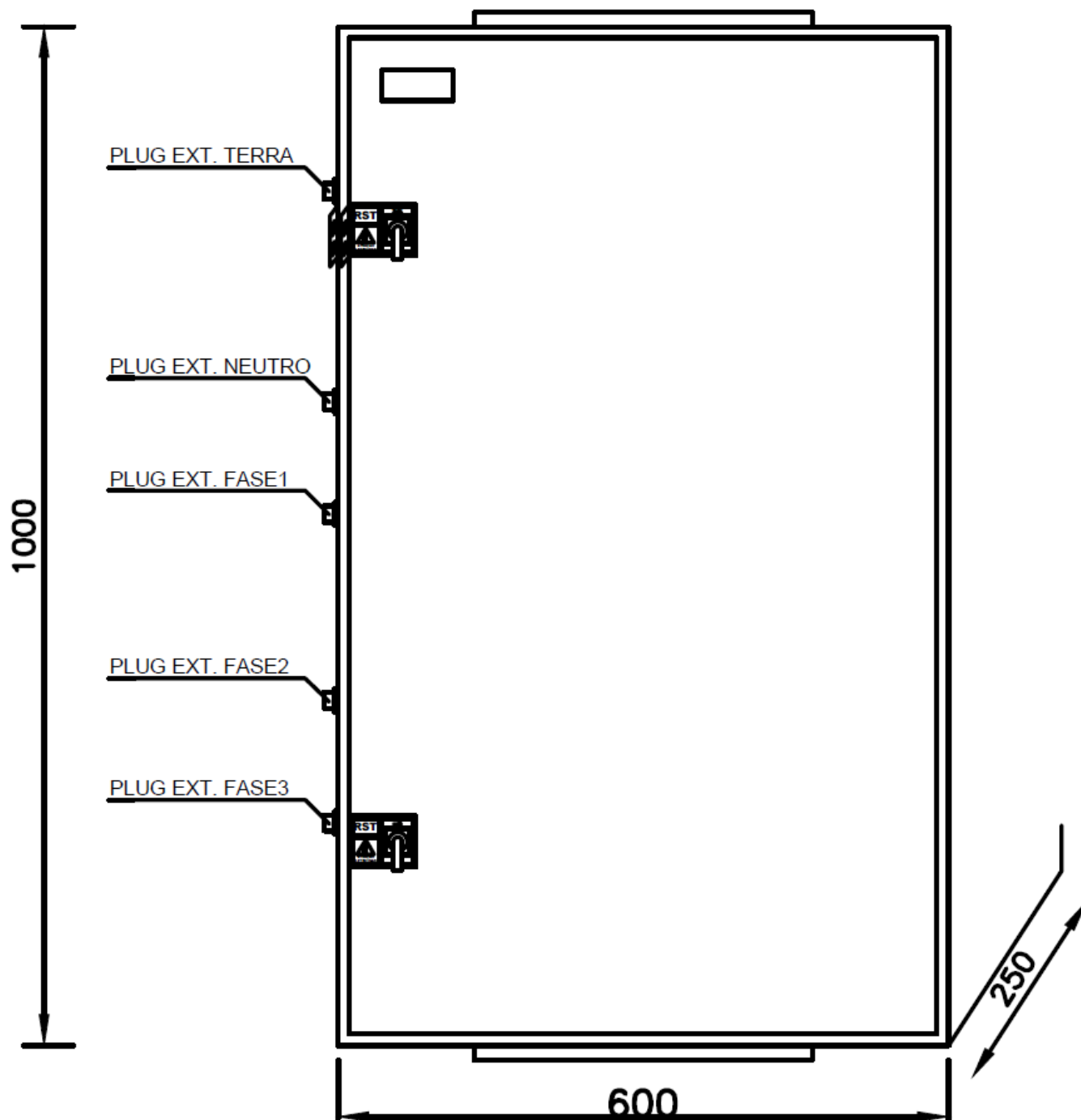
VISTA EXTERNA
