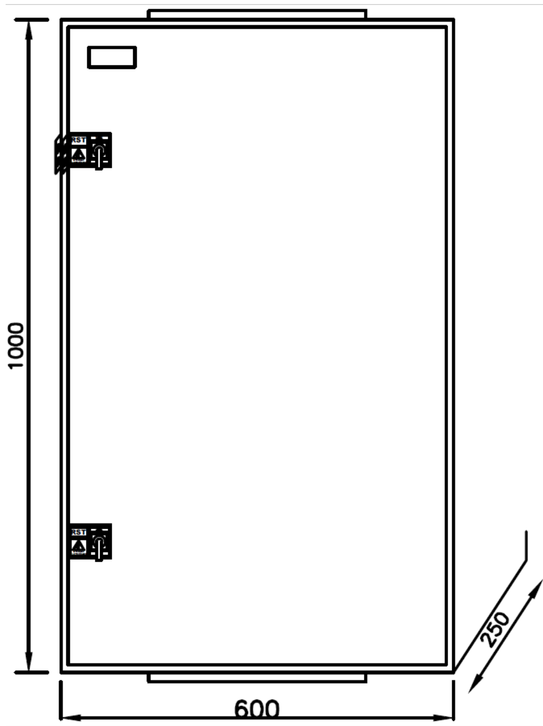
VISTA EXTERNA
