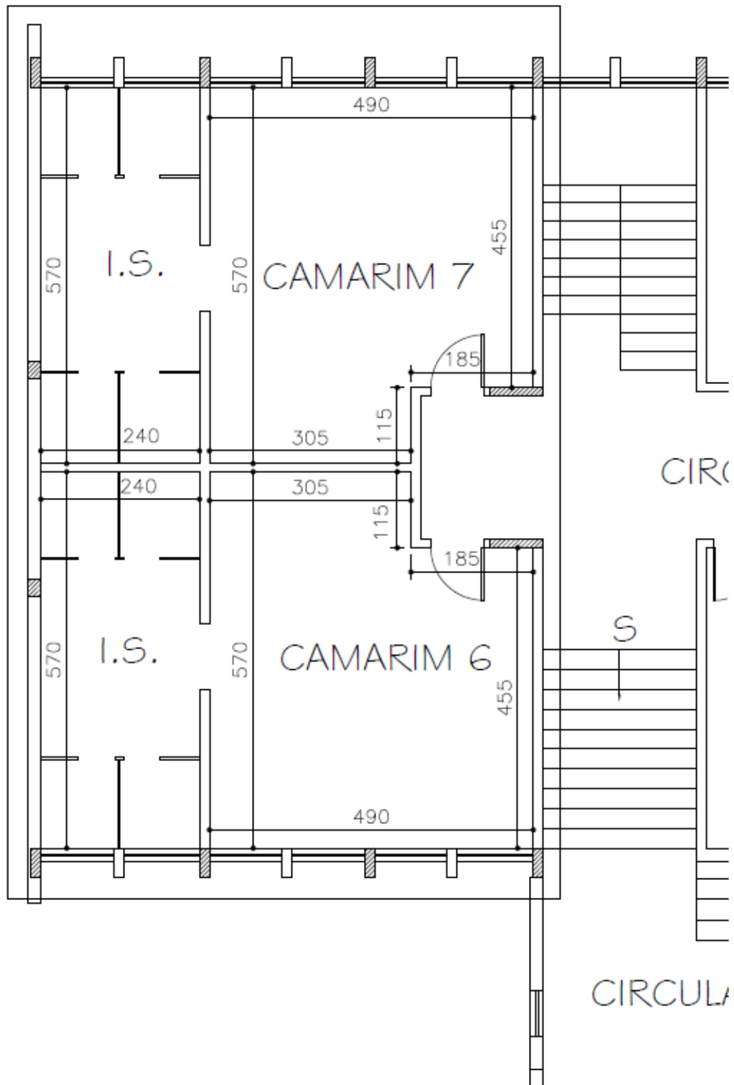
PLANTA CAMARINS NO NÍVEL INFERIOR
