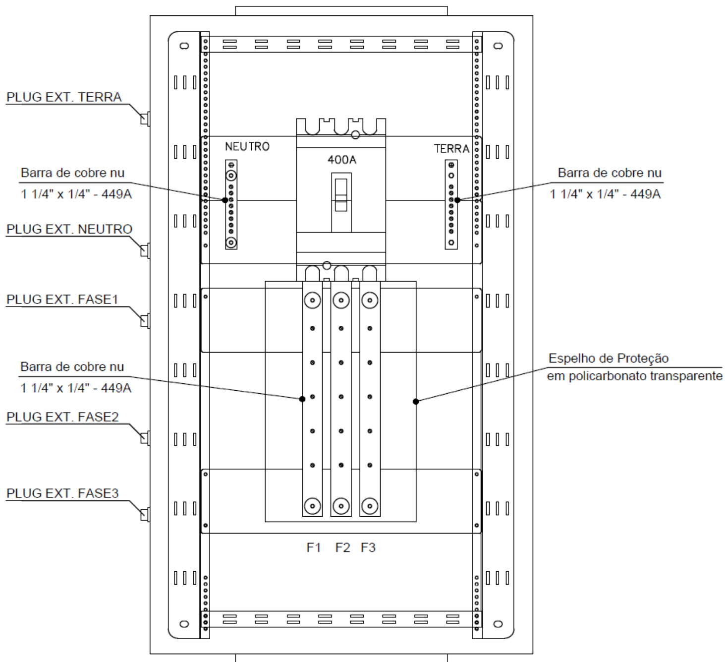
VISTA INTERNA
